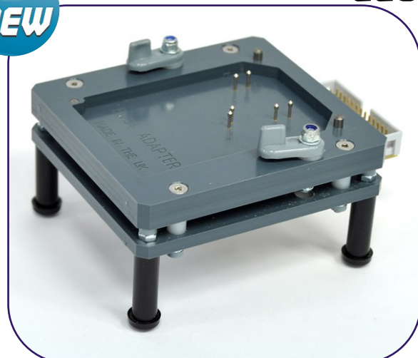
Adaptador para lectura rápida centralita EWS4 BMW.
